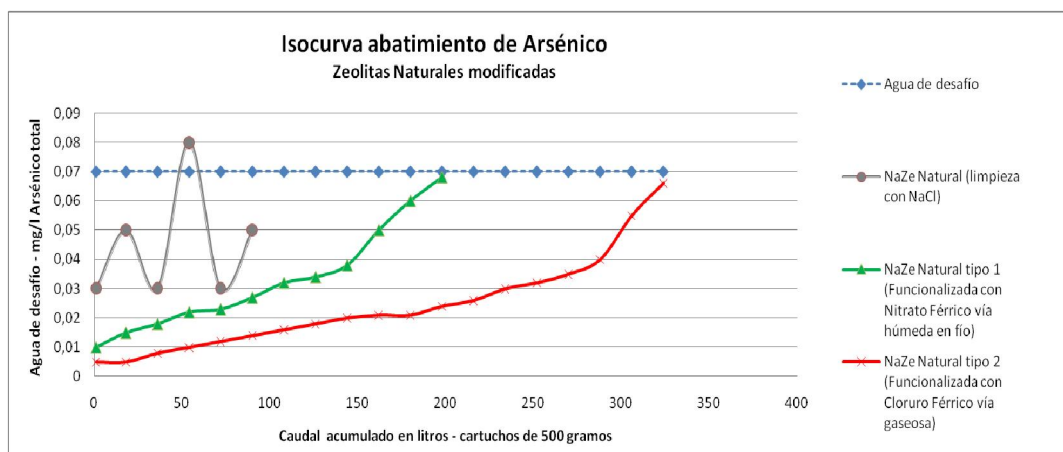
Figura 1. Isocurvas obtenidas. Velocidad de avance de lecho: 18 centímetros por minuto (100 segundos de residencia)
