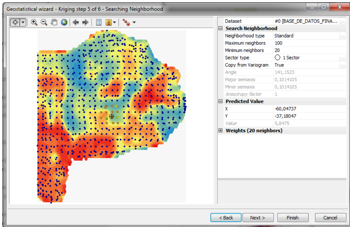
Ilustración 80 - Geostatistical Wizard: Selección de vecinos y formato de sector de búsqueda, variable "pH"
