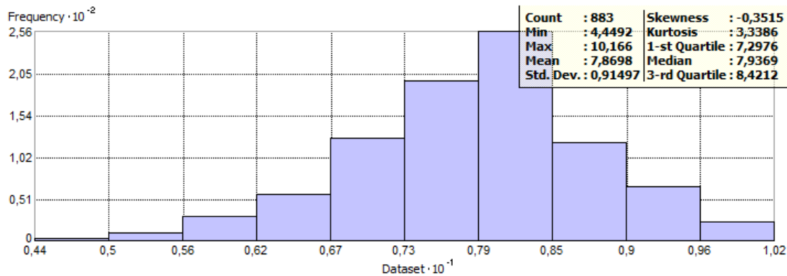
Ilustración 34 - Histograma, variable "Resistividad a 1 metro de profundidad" con transformación logarítmica"
