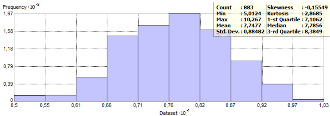
Ilustración 66 – Histograma, variable "Resistividad a 1 metro de profundidad con transformación logarítmica" sin valor atípico extremo
