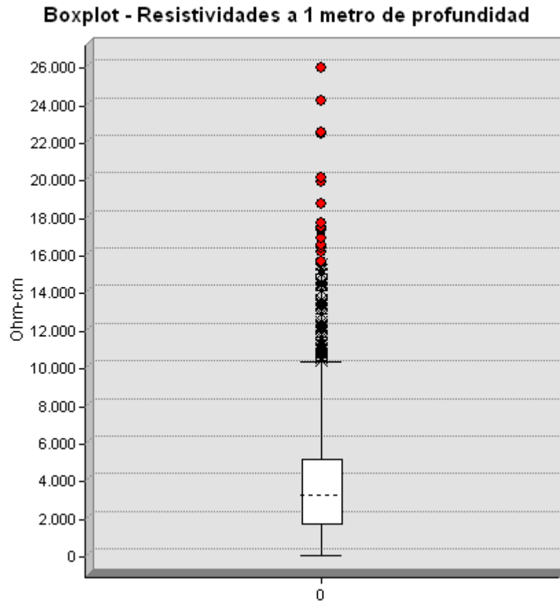
Ilustración 37 – Boxplot variable “Resistividades a 1 metro de profundidad”
