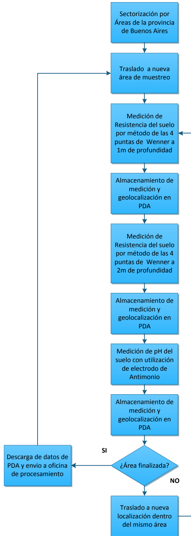
Ilustración 24 - Procedimiento de recolección de muestras
