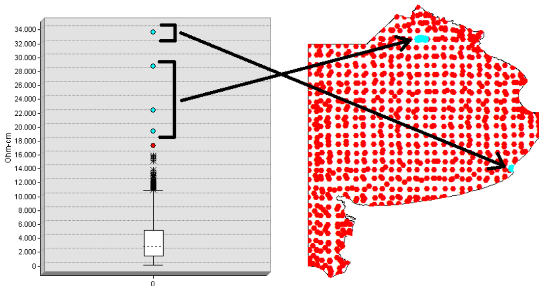
Ilustración 60 – Geolocalización de valores atípicos variable "Resistividad a 2 metros de profundidad"
