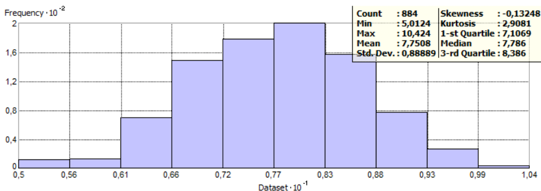
Ilustración 55 – Histograma, variable "Resistividad a 2 metros de profundidad" con transformación logarítmica
