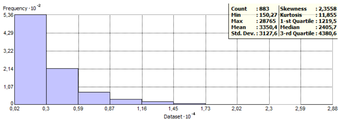
Ilustración 65 – Histograma, variable "Resistividad a 2 metros de profundidad" sin valor atípico extremo
