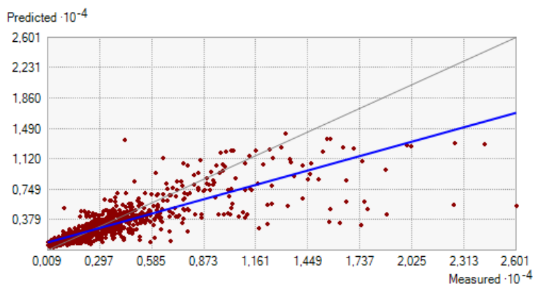
Ilustración 50 - Gráfico de valores medidos vs predicción, variable "Resistividad a 1 metro de profundidad"
