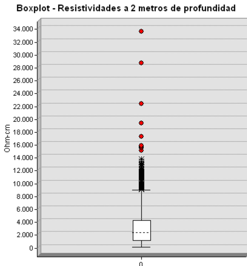
Ilustración 58 – Boxplot, variable "Resistividad a 2 metros de profundidad"
