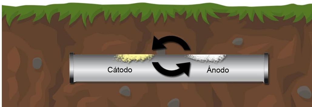
Ilustración 3 – Celda de corrosión microscópica sobre tubería - Fuente: Elaboración propia en base a NACE International cathodic protection technician
