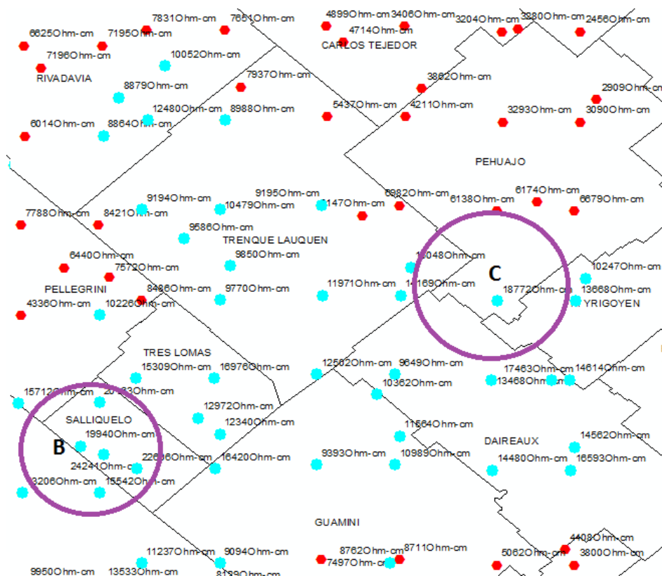
Ilustración 42 - Valores extremos de variable "Resistividad a 1 metro de profundidad" localizados en los partidos de Pehuajo y Salliquelo
