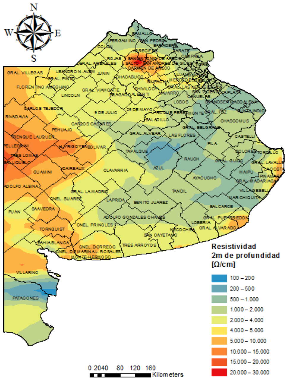
Ilustración 72 - Mapa de resistividad a 2 metros de profundidad de la Provincia de Buenos Aires
