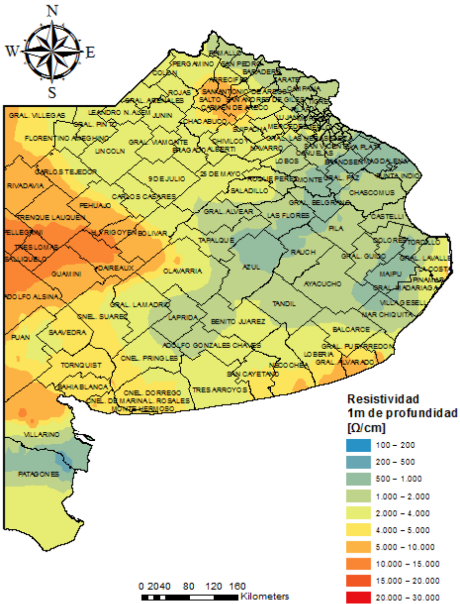
Ilustración 52 - Mapa de resistividad a 1 metro de profundidad de la Provincia de Buenos Aires
