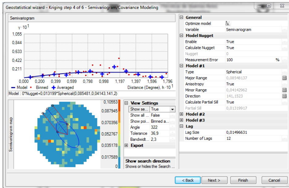
Ilustración 69 - Geostatistical Wizard: Semivariograma, variable "Resistividad a 2 metros de profundidad"
