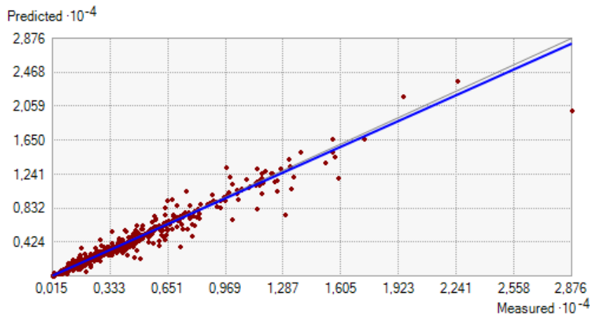
Ilustración 70 - Gráfico de valores medidos vs predicción, variable "Resistividad a 2 metros de profundidad"
