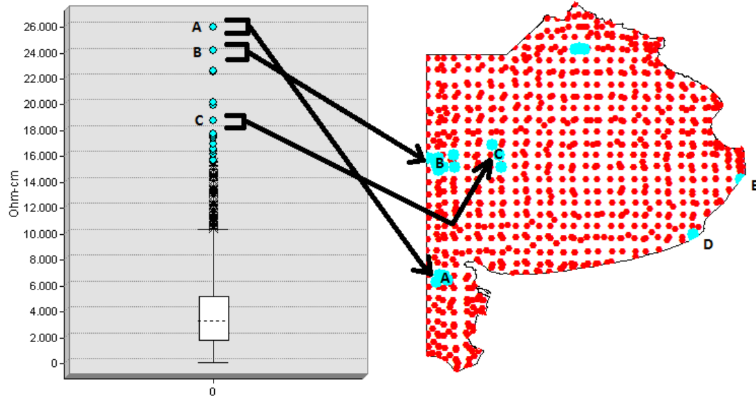
Boxplot - Resistividades a 1 metro de profundidad
