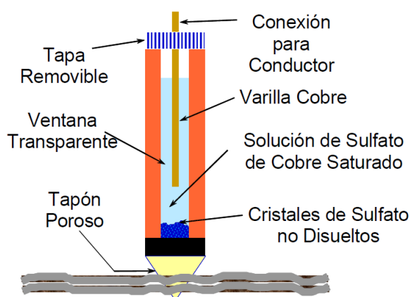
Ilustración 6 – Electrodo de referencia cobre sulfato de cobre en contacto con la tierra - Fuente: NACE International cathodic protection technician
