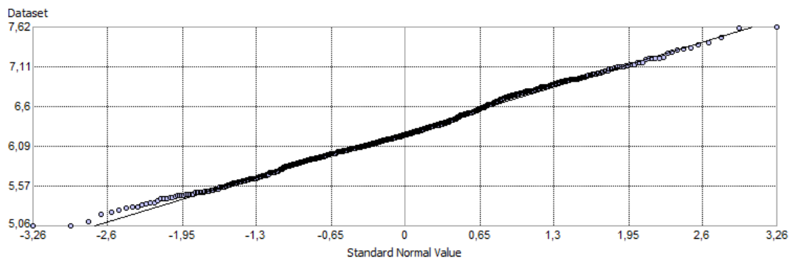
Ilustración 76 - Valor normal estándar de variable pH
