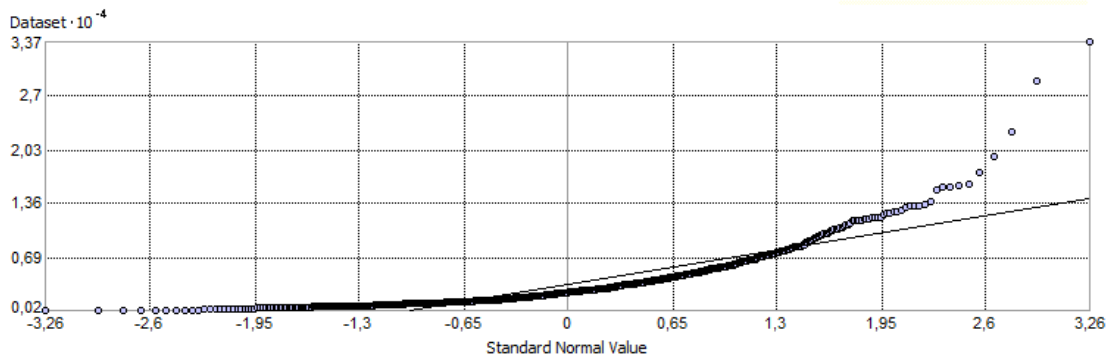
Ilustración 56 - Valor normal estándar de variable resistividad a 2 metros de profundidad
