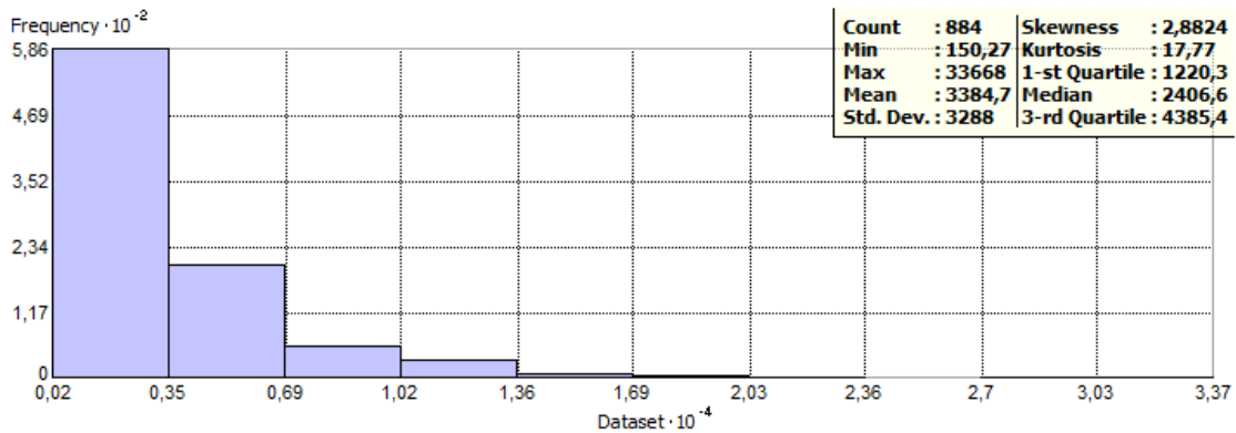
Ilustración 54 – Histograma, variable "Resistividad a 2 metros de profundidad"
