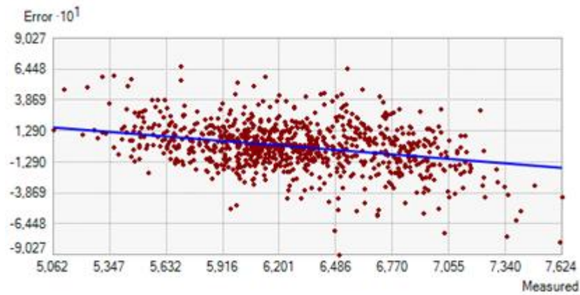
Ilustración 82 - Gráfico de valores medidos vs error, variable "pH"
