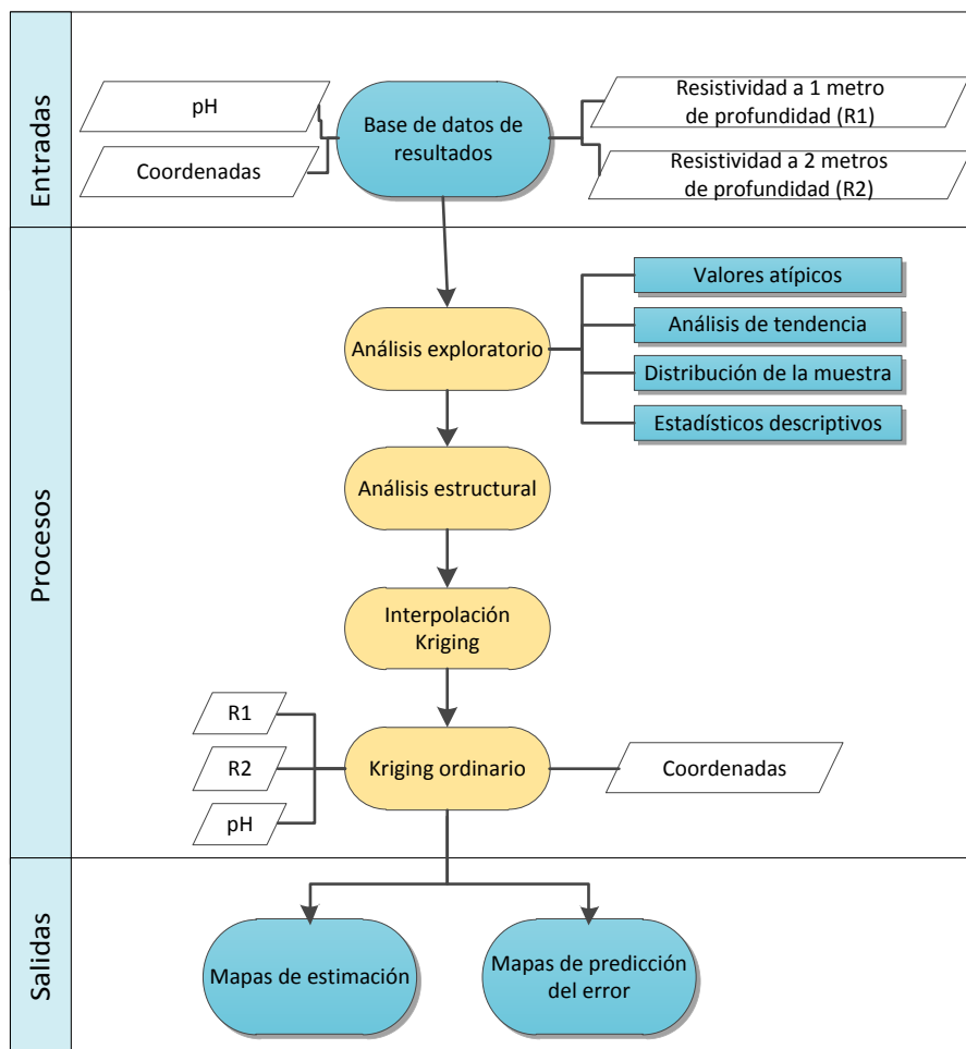
Ilustración 30 - Proceso de análisis de datos
