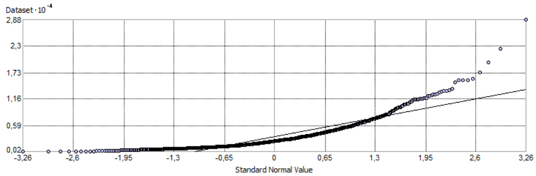
Ilustración 67 - Valor normal estándar de variable "Resistividad a 2 metros de profundidad" sin valor atípico extremo
