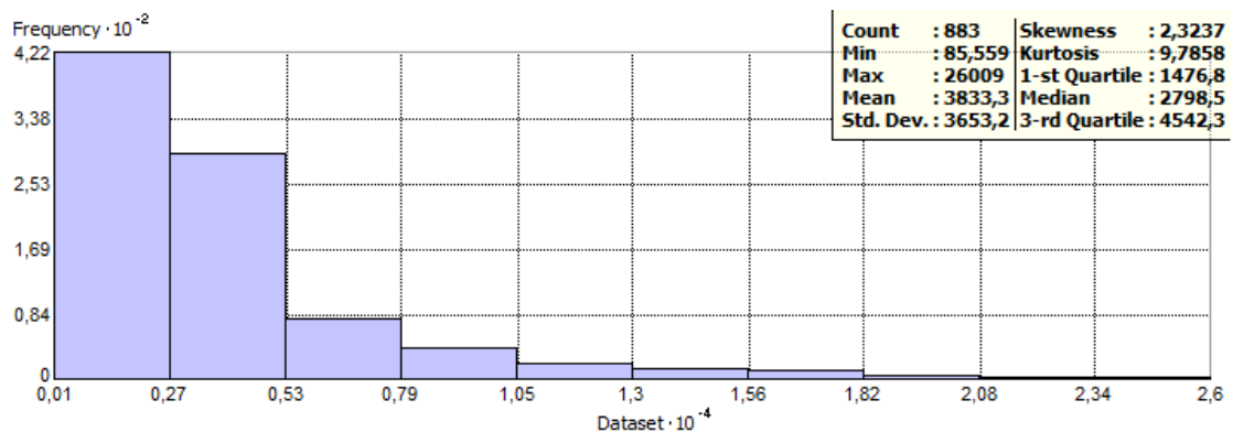
Ilustración 33 – Histograma, variable "Resistividad a 1 metro de profundidad"
