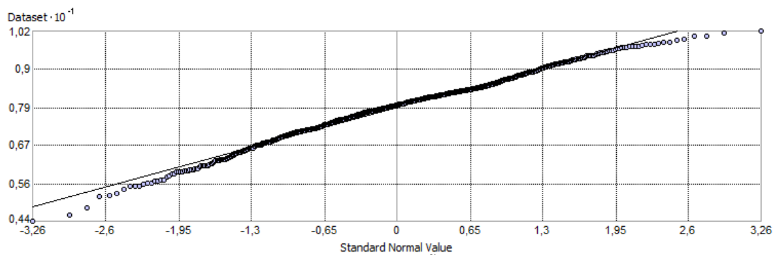
Ilustración 35 - Valor normal estándar de variable "Resistividad a 1 metro de profundidad"
