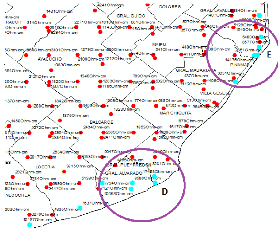
Ilustración 44 - Valores extremos de variable "Resistividad a 1 metro de profundidad" localizados en la costa de la provincia de Buenos Aires
