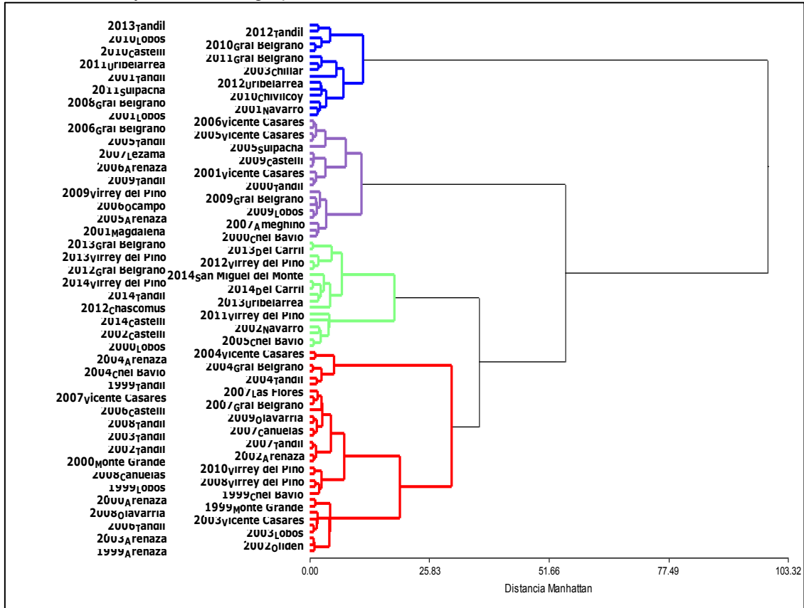
Figura 9: Fenograma clasificando ambientes para datos de lotes de producción utilizando la variable de rendimiento (materia seca, RMS) y las de calidad (digestibilidad in vitro , DIV; fibra detergente neutro, FDN; fibra detergente ácido, FDA y lignina detergente ácido, LDA) construido con manhattan y método de agrupamiento distancia mínima de Ward. CCC: 0,69.
