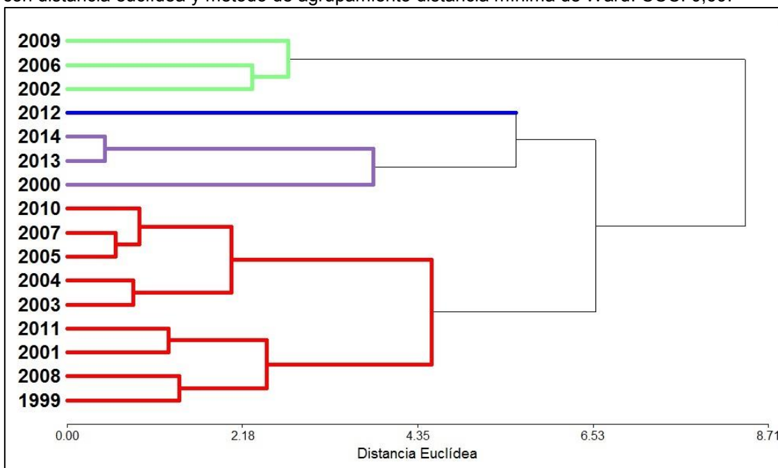
Figura 7: Fenograma clasificando los años para datos de parcelas experimentales utilizando la variable de rendimiento (materia seca, RMS) y las de calidad (digestibilidad in vitro , DIV; fibra detergente neutro, FDN; fibra detergente ácido, FDA y lignina detergente ácido, LDA) construido con distancia euclídea y método de agrupamiento distancia mínima de Ward. CCC: 0,69.
